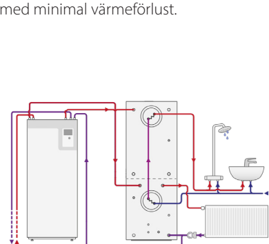
Exempelutförande bergvärmepump
