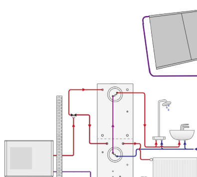
Exempelutförande luft/vatten-värmepump
